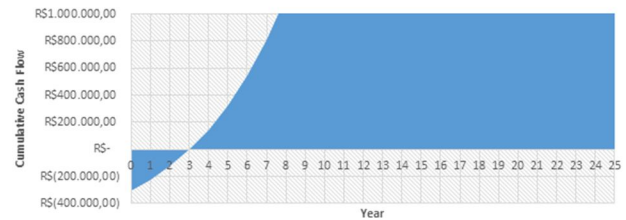
Fig. 29. Payback plot
